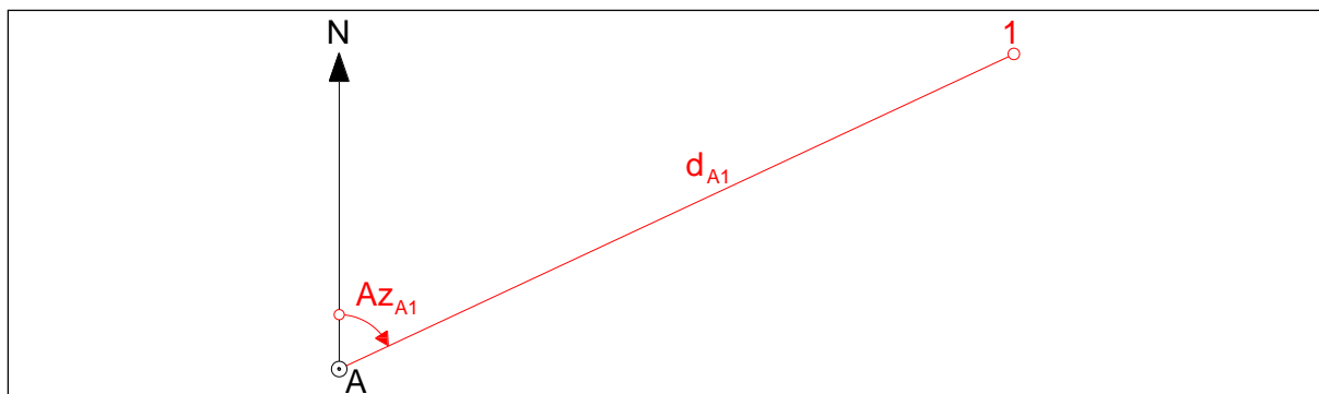
Figura 11 – Irradiação observando azimute e distância
